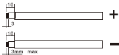
Рисунок 4 Разделка солнечного кабеля
