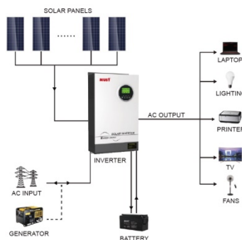
Рисунок 1 Гибридный солнечный инвертор
