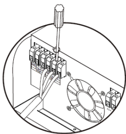
Рисунок 3 Подключение вывода переменного тока
