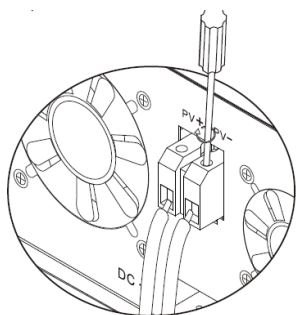
Рисунок 5 Подключение кабеля солнечных панелей
